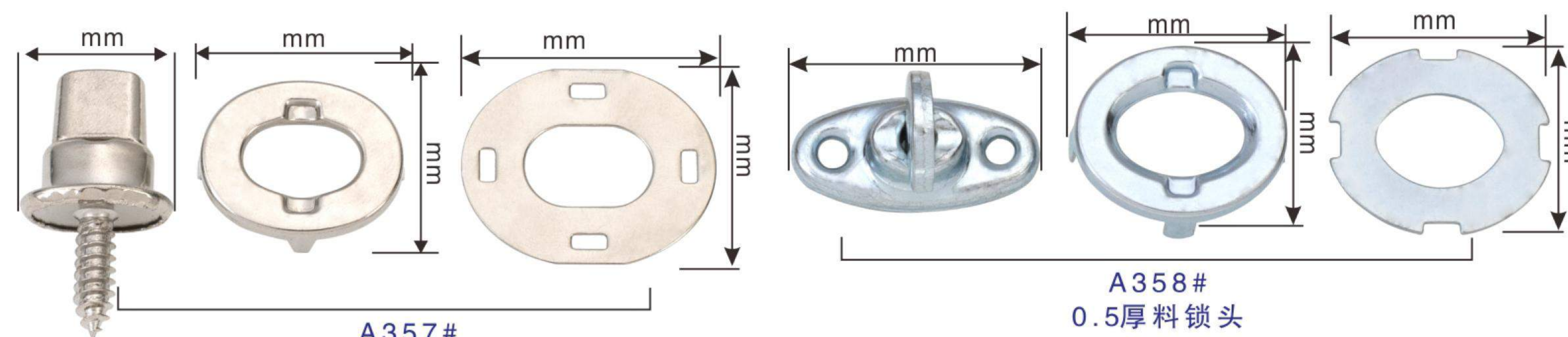
A357# 235#带螺丝锁头配平面 重量:12.5克
