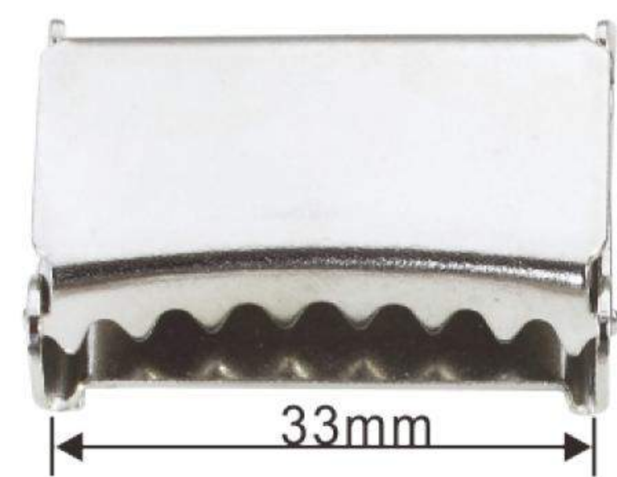
A127# 33mm调节扣 重量: 16克
