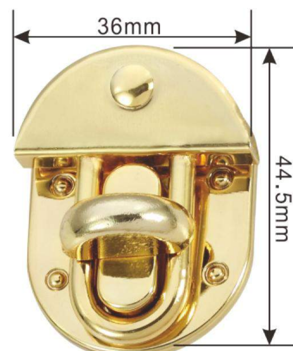
A111#半元头拧锁 重量: 23.4g
